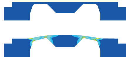
Ilustración de un sensor de acero como modelo de elementos finitos: arriba en estado despresurizado y abajo con la presión máxima.
