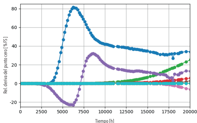
Deriva cero de sensores de película fina a 100 bar de hidrógeno
